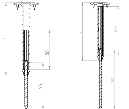
VILPE® łącznik Croco A + regulowana śruba 95. L to długość łącznika Croco.
